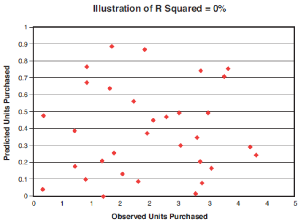
Hình 3.4. Minh họa cho đầu ra của phân tích hồi qui với r bình phương = 0
