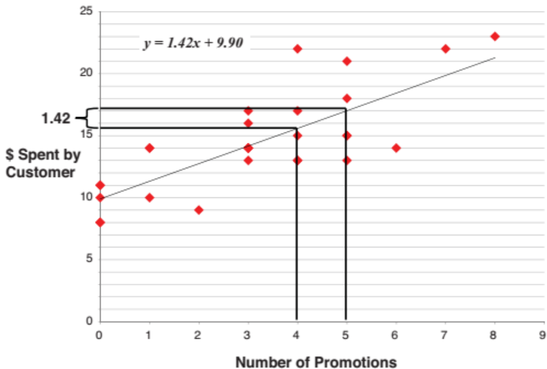
Hình 3.2. Minh họa về các thành phần trong hàm hồi qui đơn biến
